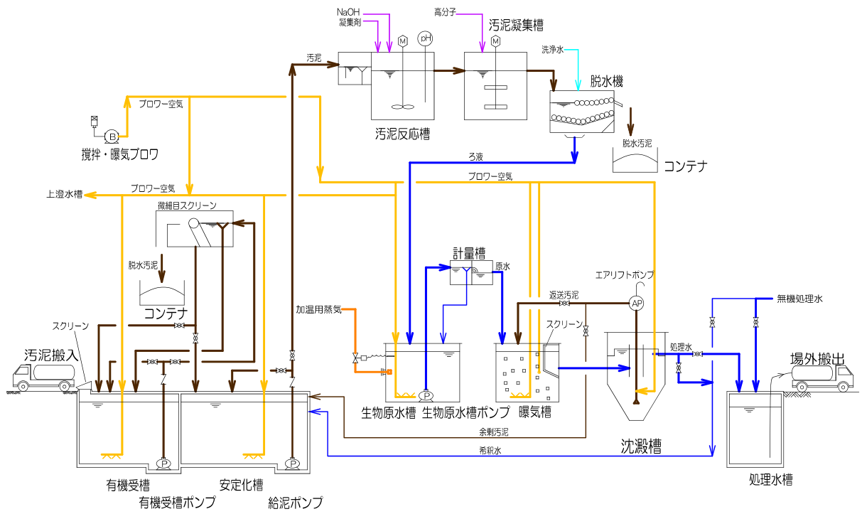
有機系汚泥処理フロー(6.086m 3 /日処理)
