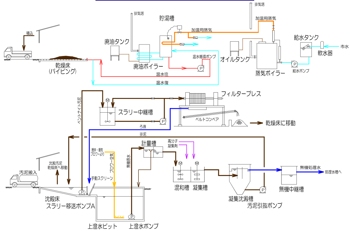
無機系汚泥処理フロー(9.990m 3 /日処理)
